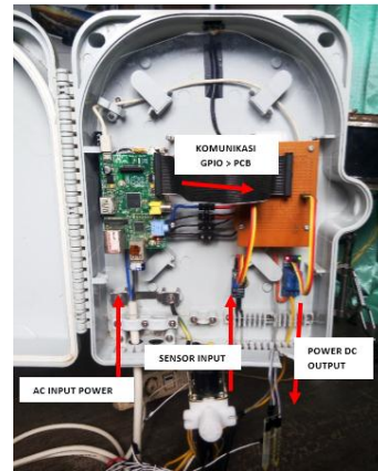
Gambar 18. Hasil Rancangan Kotak Unit Kontrol
