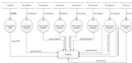
Gambar 6 Data Flow Diagram (DFD) Level 1 Pembuatan Laporan
