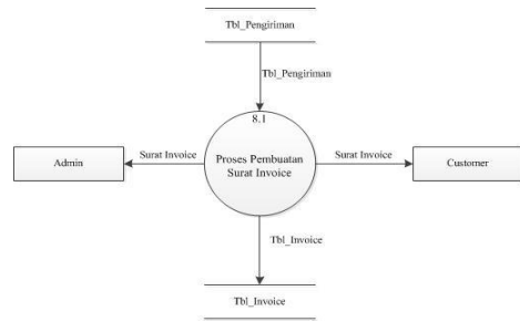
Gambar 5 Data Flow Diagram (DFD) Level 1 Pembuatan Surat Invoice
