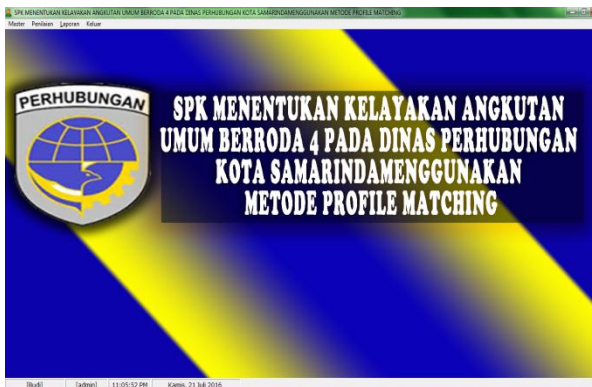
Gambar 11. Form Utama
