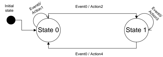
Gambar 3.1 Contoh diagram state sederhana.
